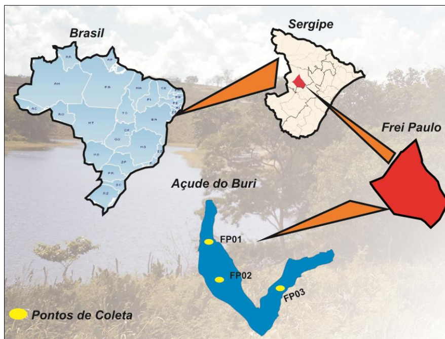
FIGURA 1a: Localização do Açude do Buri em âmbito nacional, regional e local e os pontos de coleta
